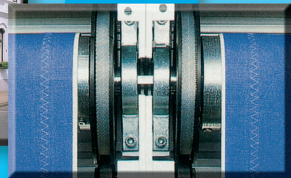
Tuchwellenkupplung für mehrteilige Markisen.
