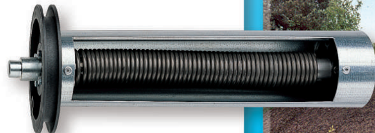
Die eingebauten Torsionsfedern sorgen bei jeder Ausfalllänge für eine optimale Tuchspannung.
